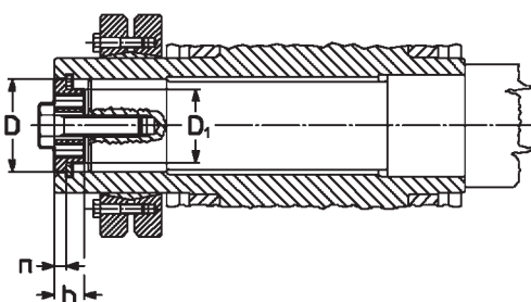
Calettamento con unità di bloccaggio c) Fitting with shrink disc c)
