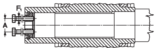
Montaggio a) e smontaggio b) Installing a) and removing b)
