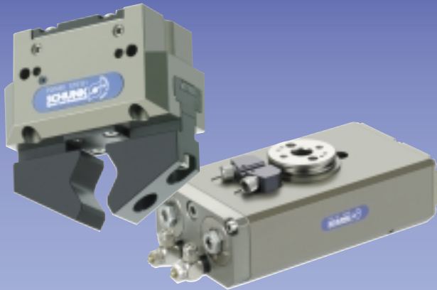
GREIFSYSTEME PNEUMATISCH
