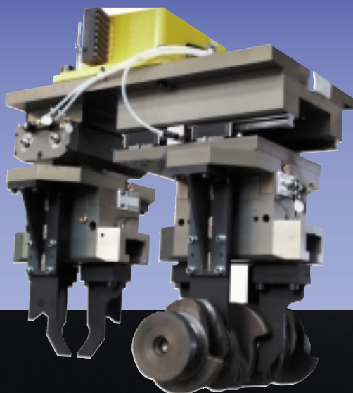
SONDERGREIFSYSTEME
